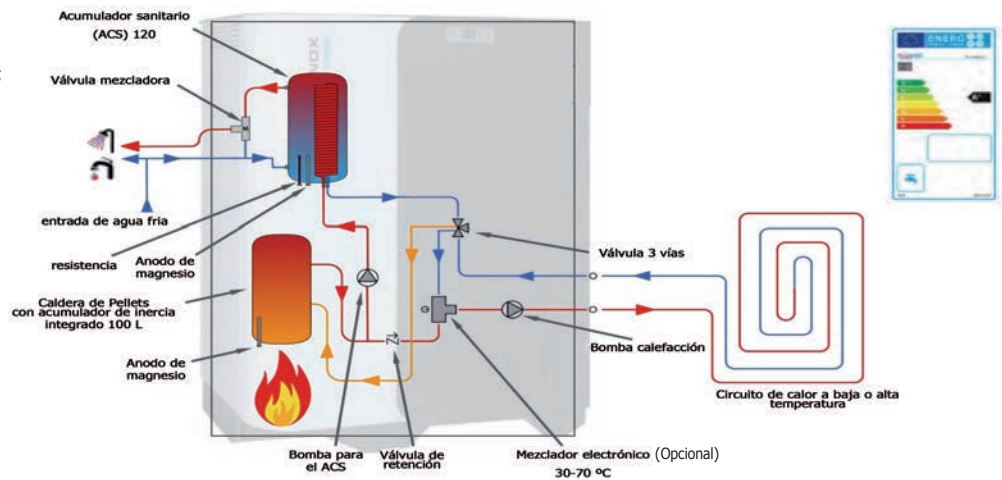
Sistema Oslo Domus combinado con acumulador ACS interno (120L)
