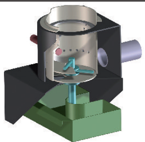
Brasero Max 24 con autolimpieza
