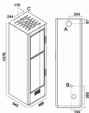
Medidas Horno Interior L300xP390xH280
